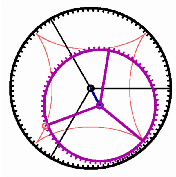
Abb. 2: Hypozykloide
