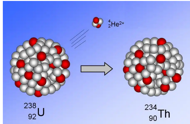
Abb. 1: Radioaktive Atomkerne zerfallen in andere Elemente, z.B. Uran in Thorium, indem sie Strahlung aussenden. Beim Alphazerfall entsteht das schwere Alpha-Teilchen aus zwei Protonen und zwei Neutronen.
