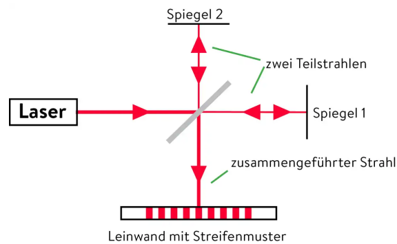
Abb. 1: Aufbau des Michelson Interferometers.
