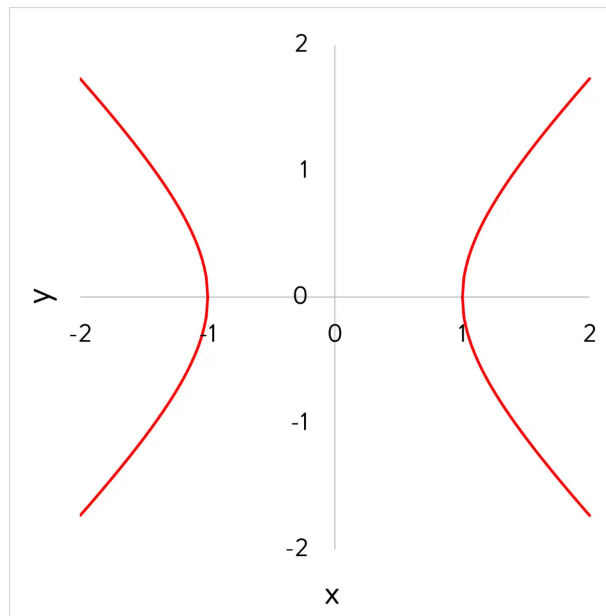
Abb. 1: Eine Hyperbel, beschrieben durch die Gleichung x^2 - y^2 = 1 .
