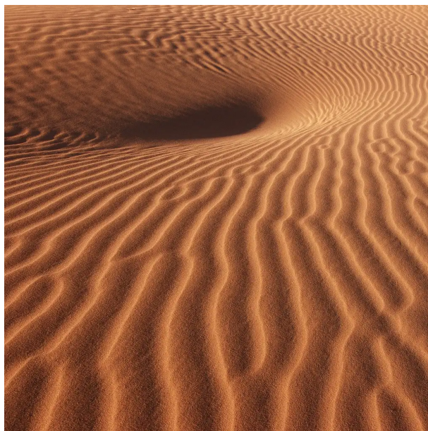
Abb. 1: Die häufigste Dünenform: Transversaldünen, langgezogene Rippel, die quer zur Windrichtung verlaufen.
