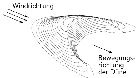
Abb. 4: Barchane wandern, indem Sand stetig vom Wind auf der flachen Seite hinaufgeweht wird und auf der anderen Seite hinunter rieselt.
